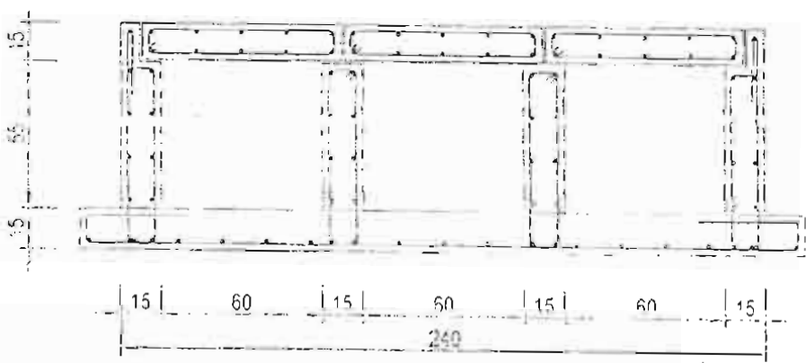
CANIVEAU TRIPLE
